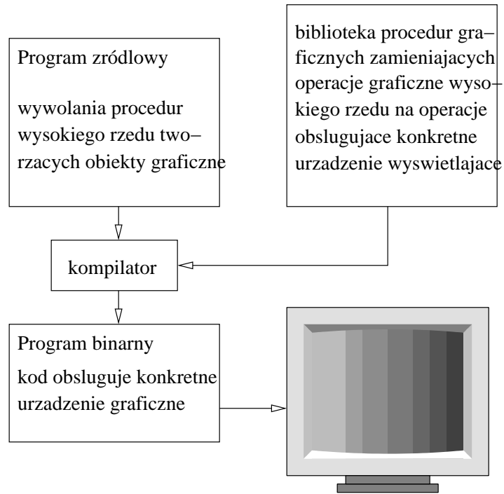
Tradycyjny schemat programu graficznego
