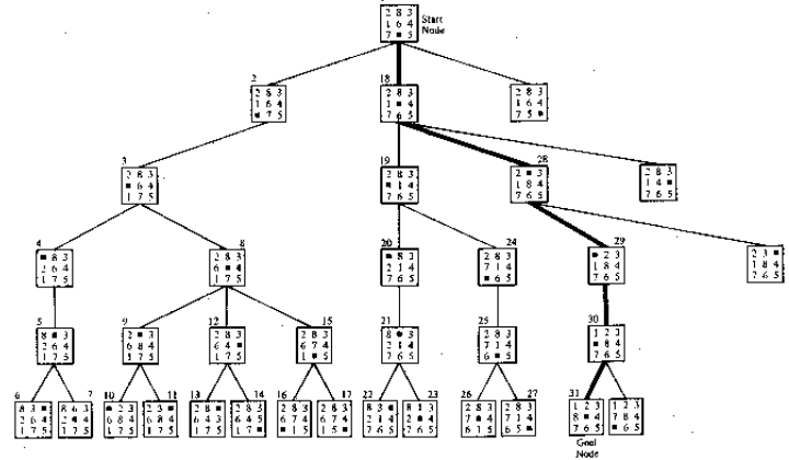
Fragment „przeciętnego” grafu przeszukiwania wgłęb z ograniczeniem głębokości do 5. Numery węzłów pokazują kolejność wyboru węzłów do ekspansji grafu.
